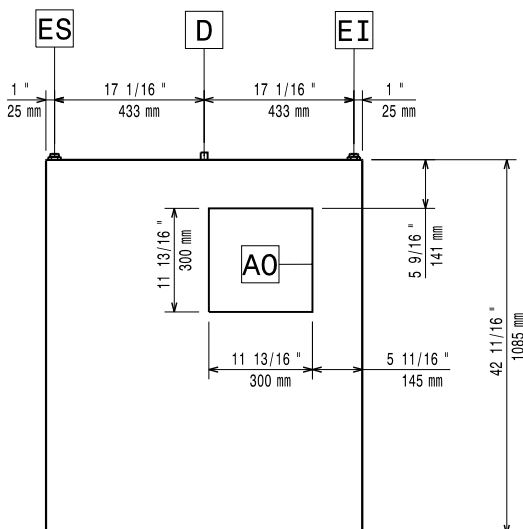
Boven aanzicht
